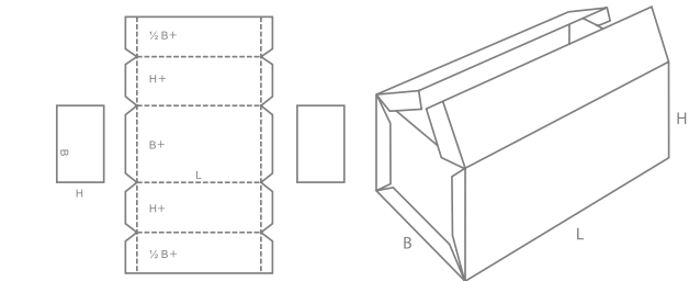
0607 | A
