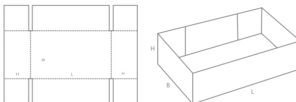
0453 | A
