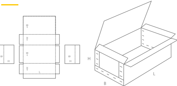
0602 | A
